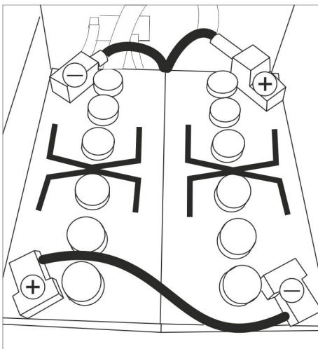
Einbauskizze für 2 Batterien
