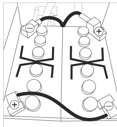
Esboço de montagem para 2 baterias
