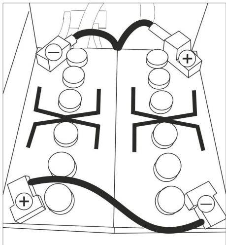
Montážní náčrsek pro 2 baterie.
