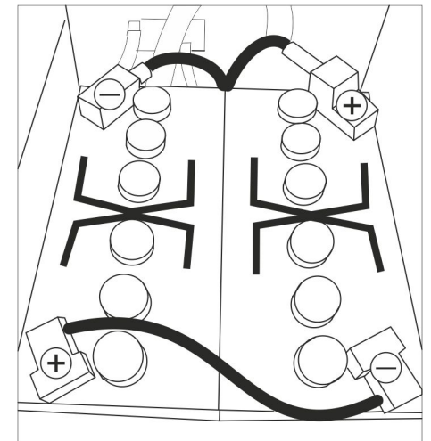
Схема встановлення для 2 акумуляторів
