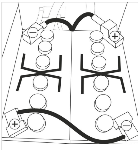
Монтажна скица за 2 акумулиращи батерии
