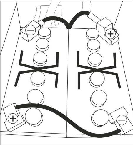
2 akü için montaj çizimi
