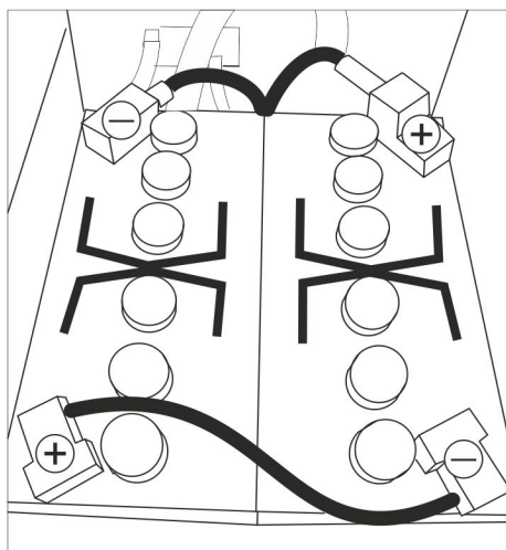
Moneringstegning for 2 batterier
